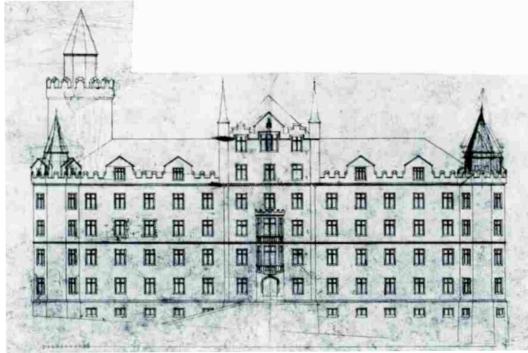
Sempers Aufriss des östlichen Hauptflügels. Mai 1842
